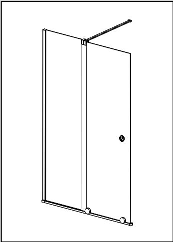
SLIDER WETROOM Rolla 8 door
