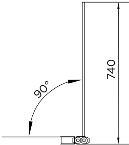
AQ6000 Square Edge Bath Screen
