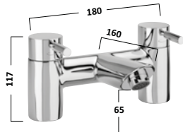
Bath Filler Chrome TKN32
