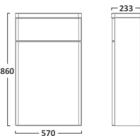
Back To Wall WC Unit Gloss White Q6BTWW Graphite Q6BTWG
